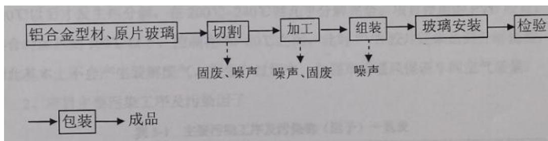
图3-9 企业生产工艺流程图
