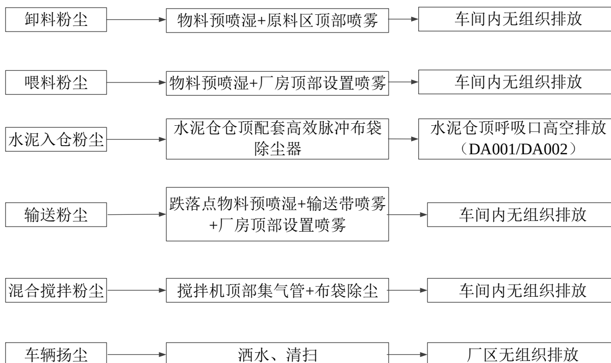
图 4-1 废气处理工艺流程图
