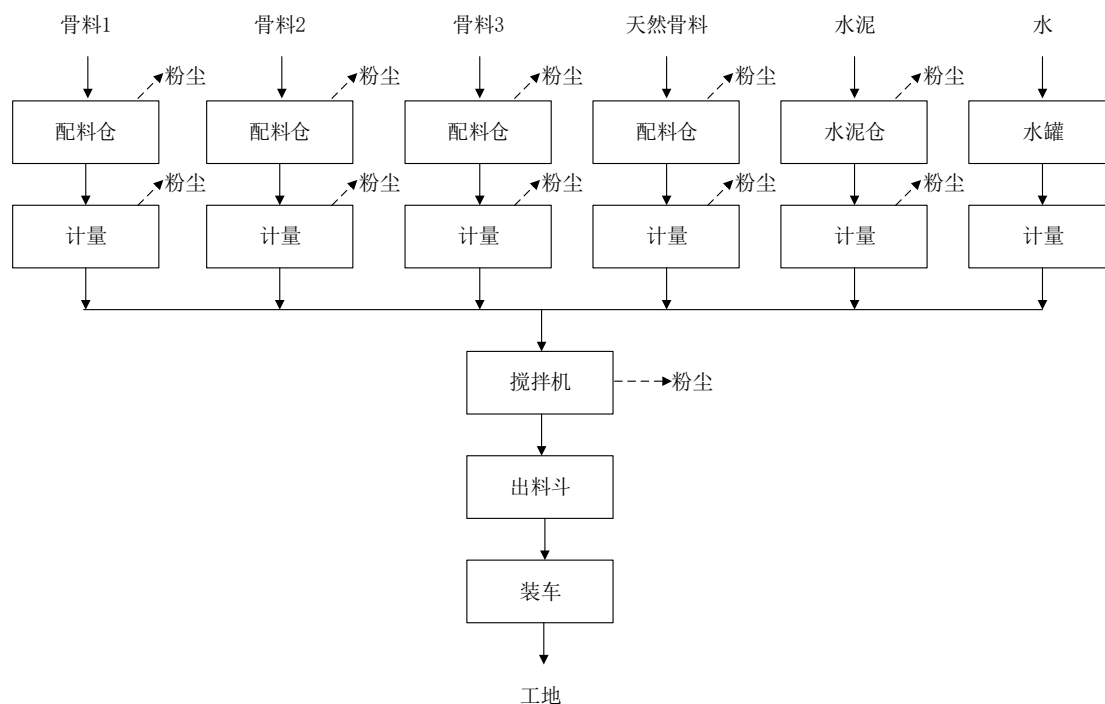
图 2-2 再生水稳层生产工艺及产污图
